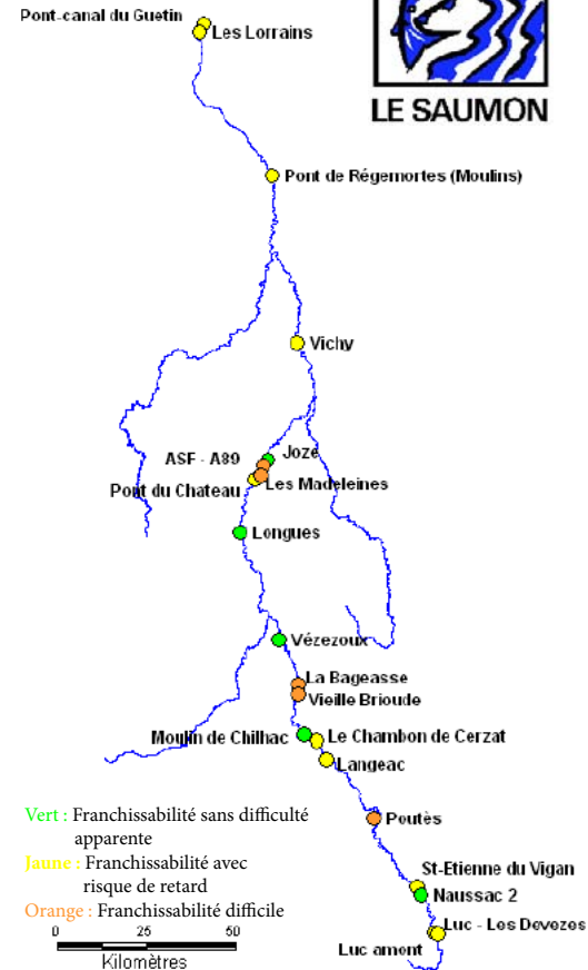
Franchissabilité des ouvrages de l'Allier à la montaison, 2012. © ONEMA
